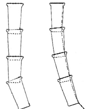
falsch (ohne Führungsseil) Skizze 6.1
