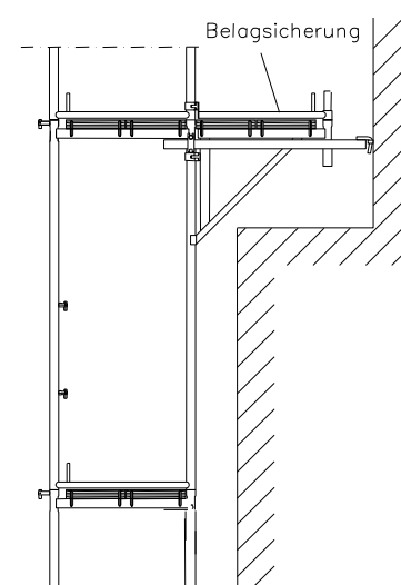
Bild 24: Konsole 64
