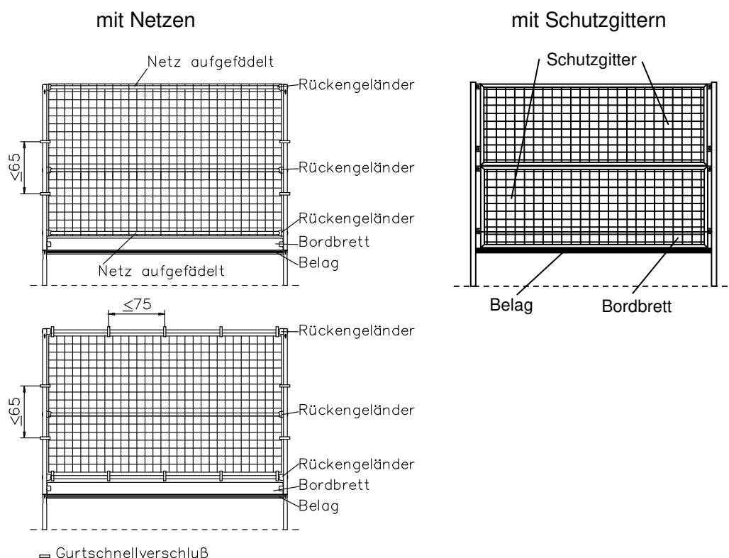
Bild 28: Schutzwand
