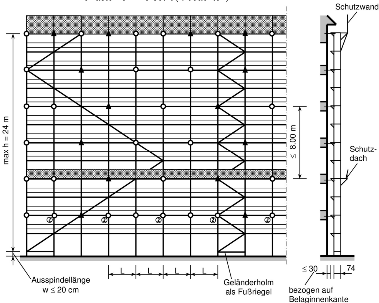
Bild 37: Konsolvariante 2 (Schutzdach in + 8 m oder höher) Ankerraster: 8 m versetzt (Ⓜbeachten)
