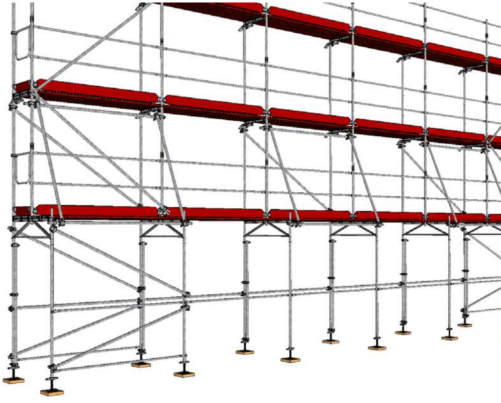
Bild 53: Durchgangsrahmen
